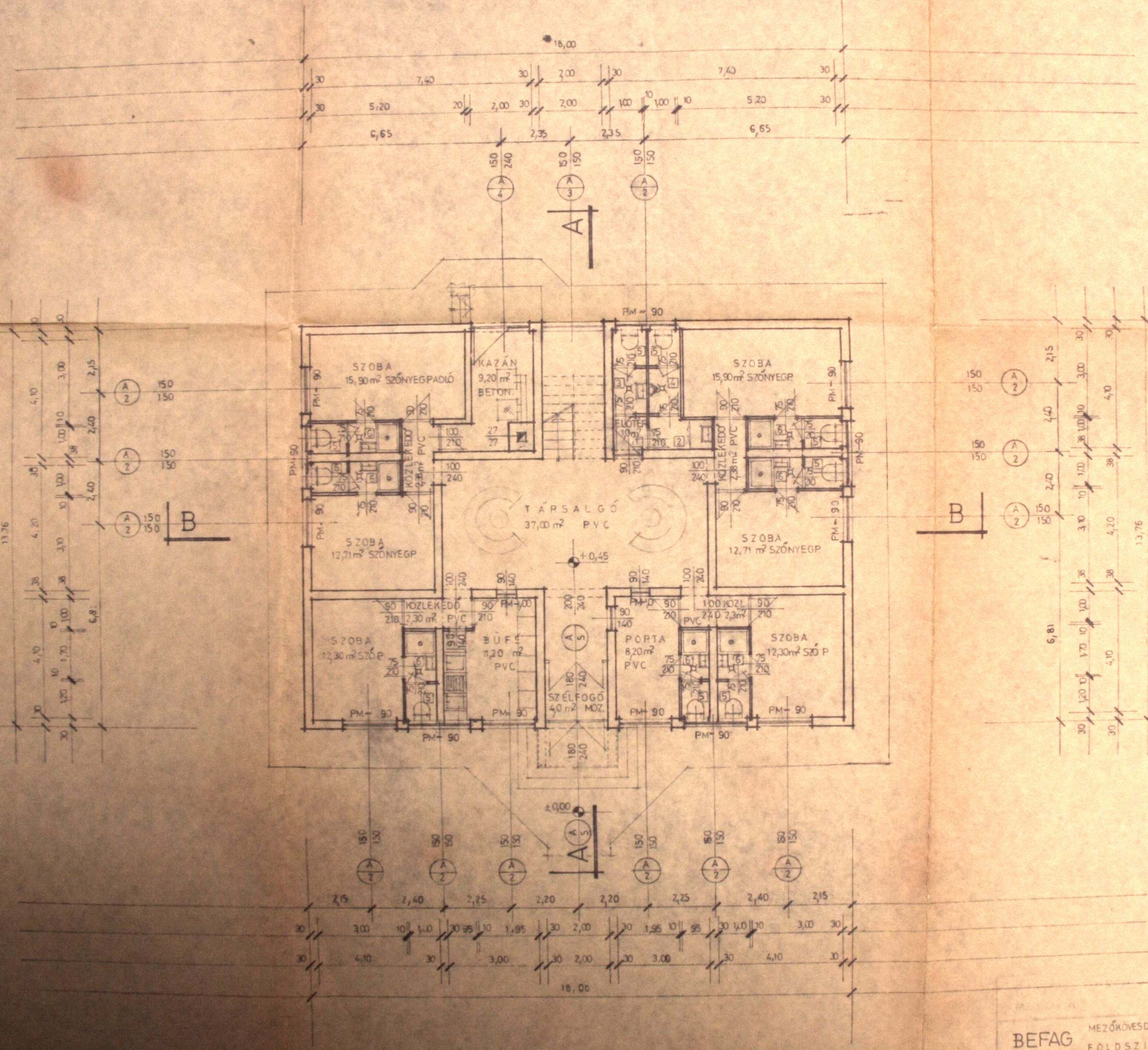
földszinti alaprajz m = 1:100
